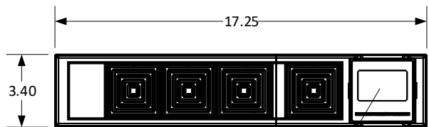
LCD Display
